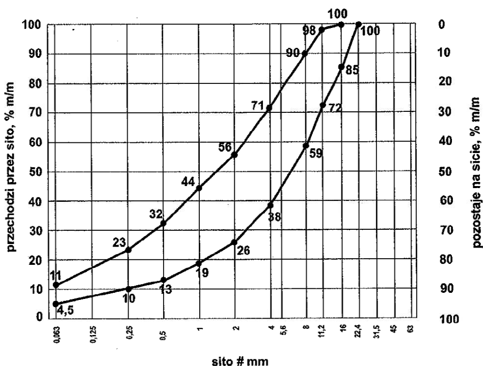
Rys. 1 Uziarnienie mieszanki CBGM 0/16 mm
