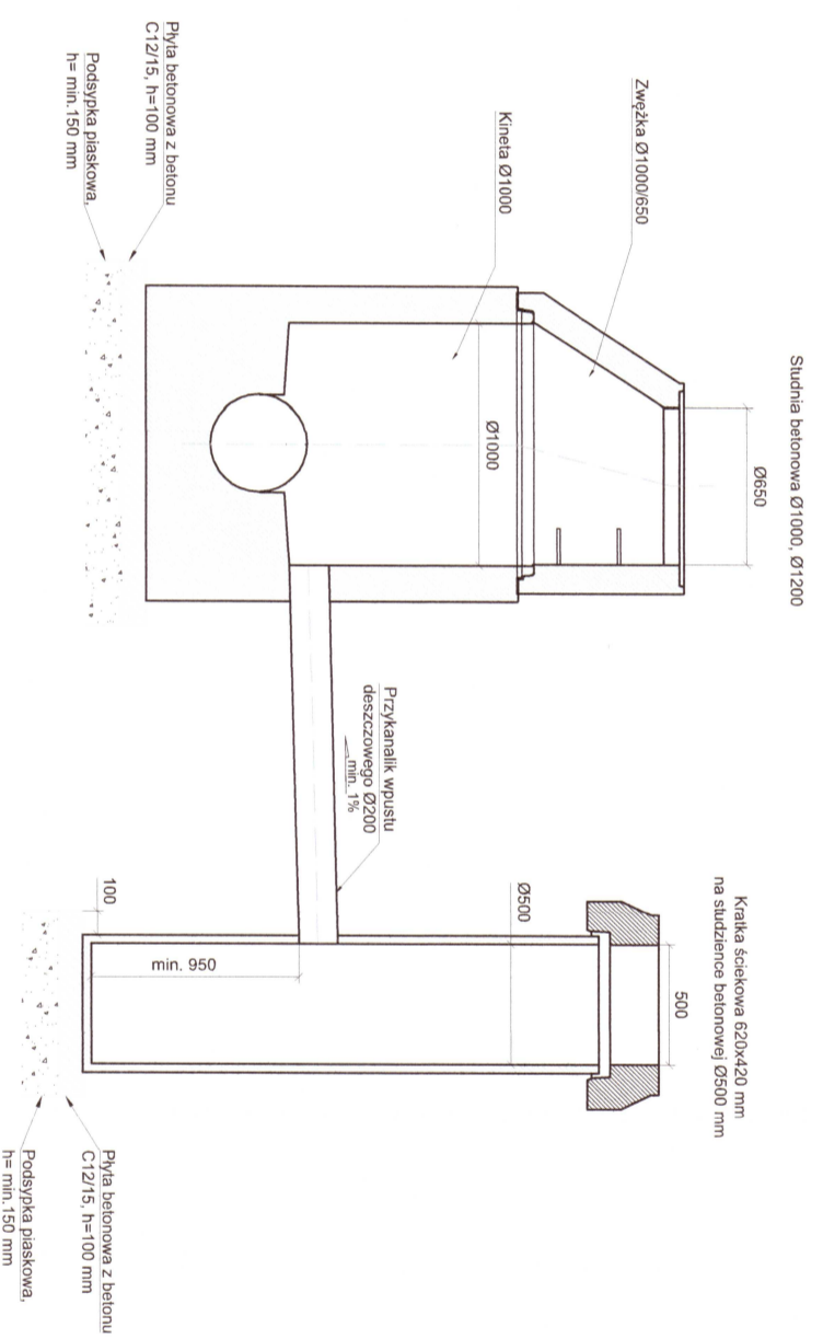
Studnia betonowa Ø1000, Ø1200
